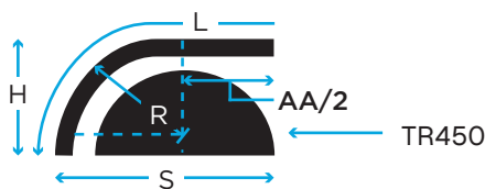
L'aile tandem est composée de 2x TR450
