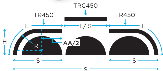
L'aile tridem JTR450 est composée de 2x TR450 et de 1x TRC450
